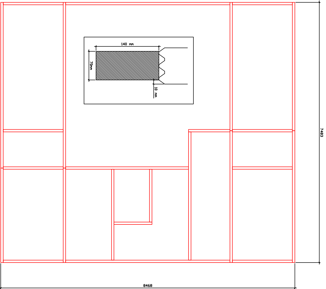
Grundplan
